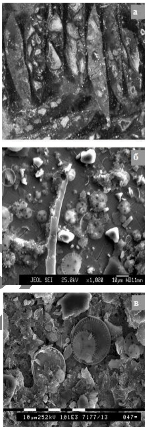
Рис.1 Изображение в оптическом микроскопе (а) поверхности брикетного шлифа с диатомовыми водорослями из Байкала; изображение во вторичных электронах высушенных на подложках каплей со створками диатомовых водорослей из озера Хубсугул, полученное при увеличении 1000-крат с помощью микро-анализатора JXA8200 (б) и электронного микроскопа Quanta 200 (в).
