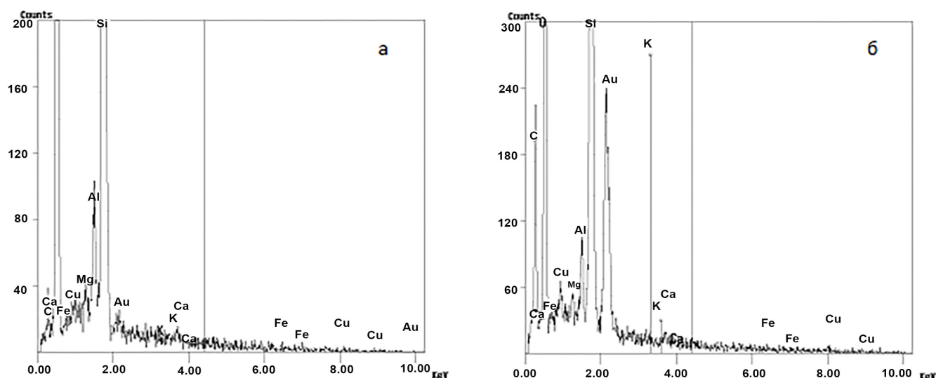
Рис.3 Рентгеновские спектры, зарегистрированные от створки диатомовой водоросли типа Cyclotella ocellata из озера Хубсугул при разных условиях измерения: а – ускоряющее напряжение E_0=10\text{ kV} , ток зода i_b=2\text{ nA} ; б – E_0=10\text{ kV} , i_b=20\text{ nA} .
