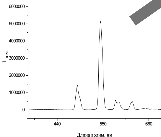
Рис. 1. Спектр люминесценции иона \text{Tb(III)} в комплексе с \alpha -горькими кислотами ( C_{\text{Tb}} = 1 \cdot 10^{-4} \text{ моль/л} ).
