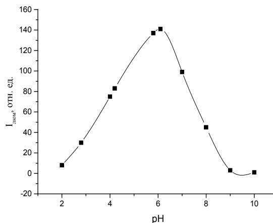
Рис. 2. Зависимость I_{\text{люм.}} иона \text{Tb(III)} в комплексе с \alpha -горькими кислотами от pH раствора ( \lambda_{\text{изл. Tb}} = 545 \text{ нм} ; C_{\text{Tb}} = 1 \cdot 10^{-4} \text{ моль/л} ).
