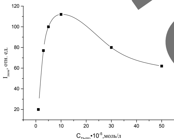
Рис. 5. Зависимость I_{\text{люм.}} иона Tb(III) в комплексе с \alpha -горькими кислотами от концентрации Tb(III) ( \lambda_{\text{изл. Tb}} = 545 \text{ нм} ).
