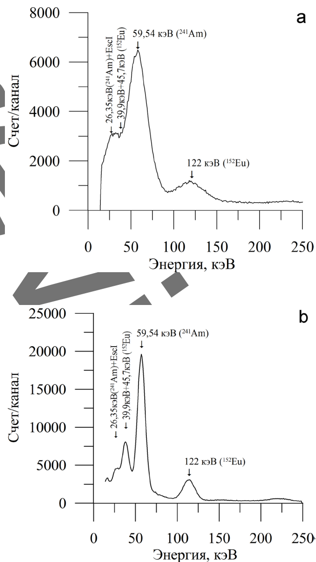
Рис.1. Спектр от радиоактивных источников ^{241}\text{Am} + ^{152}\text{Eu} : а) БД БДЭГ2-39-01; б) БД БДЭГ2-38.
