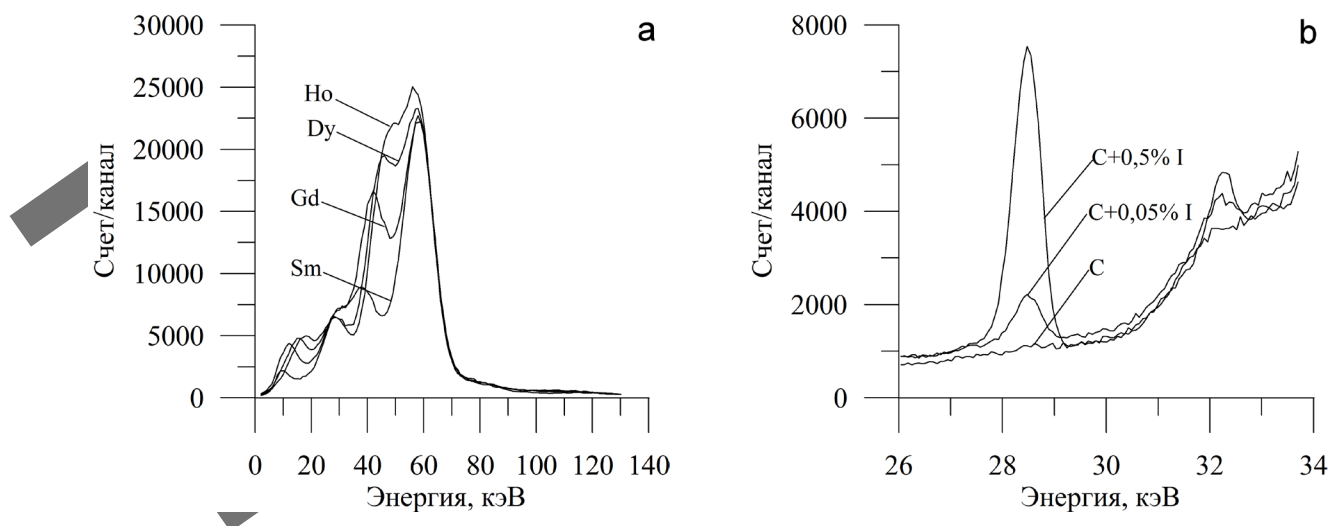
Рис. 3. Спектры х.р.и.от градуировочных образцов, измеренные БД XR100T AMPTEK при возбуждении источником ИГИА-1м-5: а) с ВИ из окиси самария; б) с ВИ из окиси церия.
