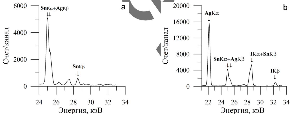
Рис. 4. Спектры х.р.и. градуировочных образцов, измеренные БД XR-100CR AMPTEK: а) аморфный углерод при одновременном облучении тремя источниками ИГИА-1м-5; б) углерод с 0.5 мас.% йода при облучении одним источником ИГИА-1м-5.
