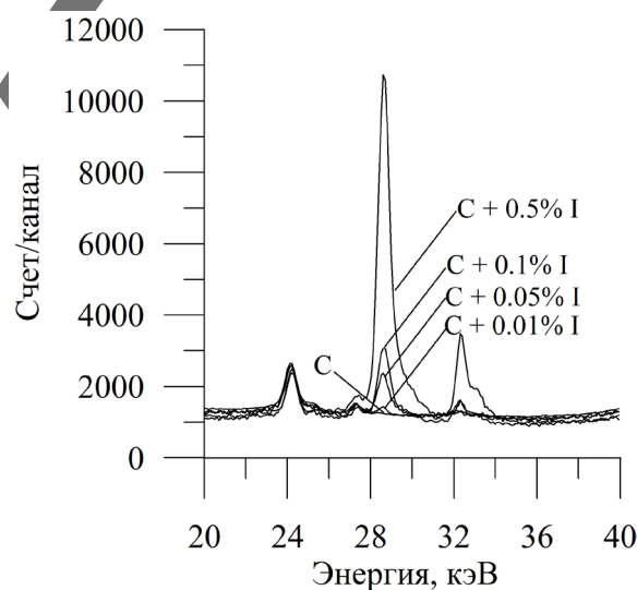
Рис.6. Спектры х.р.и. градуировочных образцов с различной массовой долей йода в углеводе и особочистого углерода при облучении источником ИГИА-1м-5, полученные с использованием БД с кристаллом Ge(HP).
