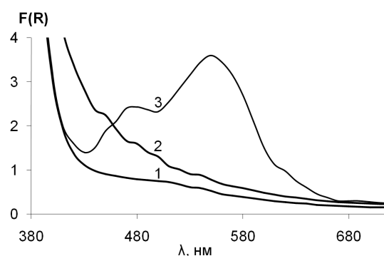
Рис. 10. СДО сорбента АБТС ( C_{\text{Pt}} , мкг/0.1 г: 0 (1), 25 (2,3), после обработки 3 \cdot 10^{-5} М ТКМ (3)).
