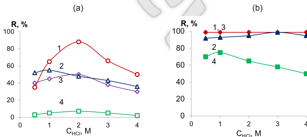
Рис. 5. Зависимости степени извлечения Ru(IV) (1), Os(IV) (2), Rh(III) (3), Ir(IV) (4), сорбентом МФС от концентрации HCl без (а) и в присутствии (б) SnCl_2 ( C_M = 2.5 мг/мл; V = 10 мл; C(SnCl_2) = 0.025 М (б); 0.1 г сорбента; время контакта фаз 30 мин; T = 95^\circ C ).
