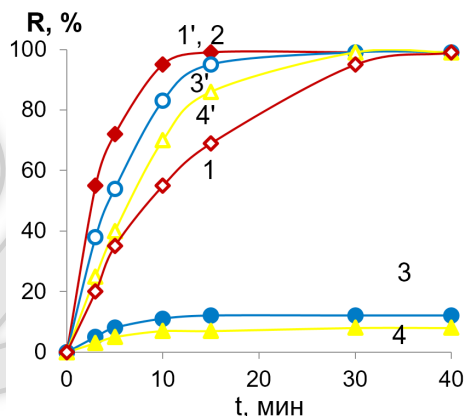
Рис. 4. Зависимости степени извлечения Au(III) (1, 1'), Pd(II) (2), Pt(II) (3, 3'), Pt(IV) (4, 4') сорбентом АБТС от времени контакта фаз ( C_M = 2.5 мкг/мл; V = 10 мл; T, ^\circ\text{C} : 95 (1-4), 25 (1', 3', 4'); 0.1 г сорбента).
