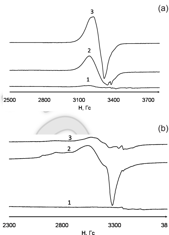
Рис. 9. Спектры ЭПР комплексов рутения, образующихся на поверхности сорбентов МФС (а), АБТС (б) в процессе сорбции из 1 М НСl в присутствии \text{SnCl}_2 (1,2) и в отсутствие \text{SnCl}_2 (3) ( C_{\text{Ru}}=100 мкг/0.2 г; время выдерживания образцов после сорбции, ч: 0 (1,3), 24 (2)).
