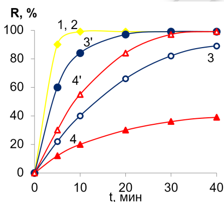
Рис. 2. Зависимости степени извлечения Au(III) (1), Pd(II) (2), Pt(II) (3, 3'), Pt(IV) (4, 4') сорбентом МФС от времени контакта фаз ( C_M = 2.5 мкг/мл; V = 10 мл; 0.1 г сорбента; T, ^\circ\text{C} : 25 (1-4), 95 (3', 4')).
