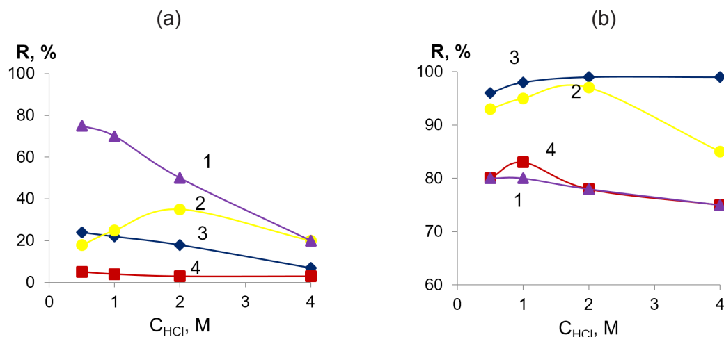
Рис. 6. Зависимости степени извлечения Os(IV) (1), Ru(IV) (2), Rh(III) (3), Ir(IV) (4) сорбентом АБТС от концентрации HCl без (а) и в присутствии (б) SnCl 2 (C M = 2.5 мкг/мл; V = 10 мл; C(SnCl 2 ) = 0.025 М (б); 0.1 г сорбента; время контакта фаз 30 мин; T = 95 °C (а,б)).
